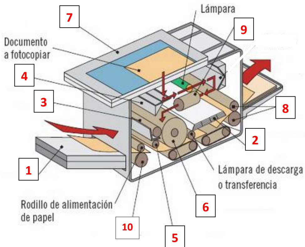
Esquema de las partes físicas de una fotocopiadora
