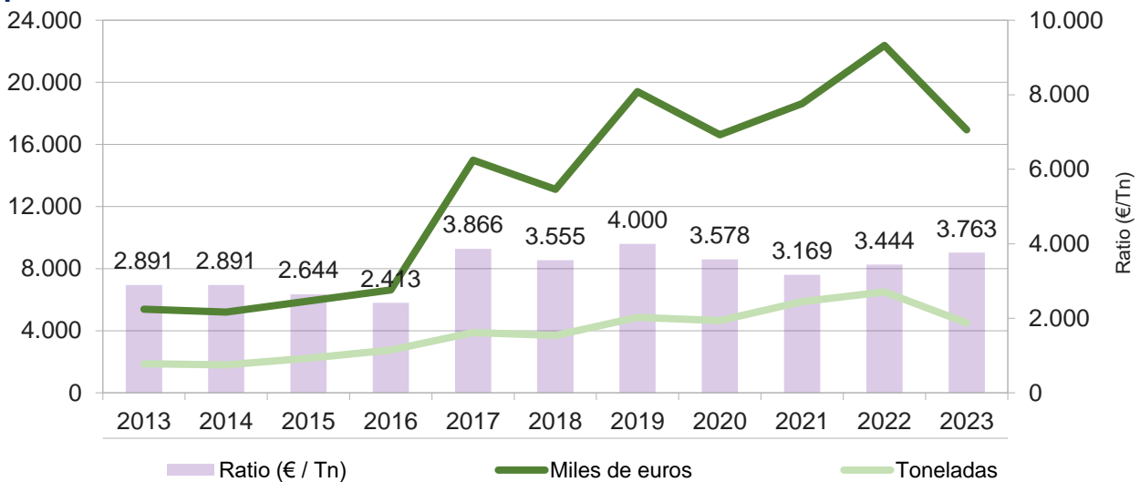
Gráfico 15: Evolución de las ventas de Corcho natural en bruto, desperdicios o corcho pulverizado a Francia.
